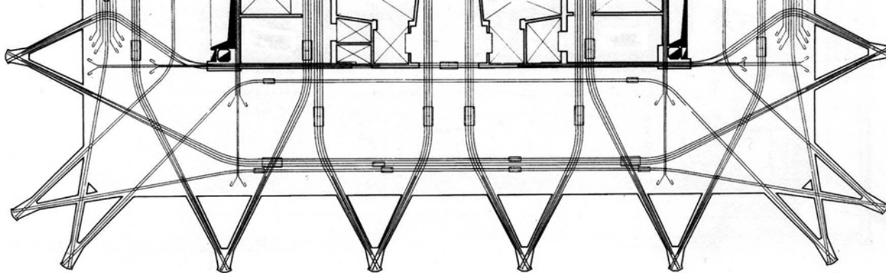
BBPR, pianta struttura 19° p. Torre Velasca, 1958
